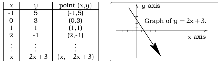
(a) Tabulated data.
