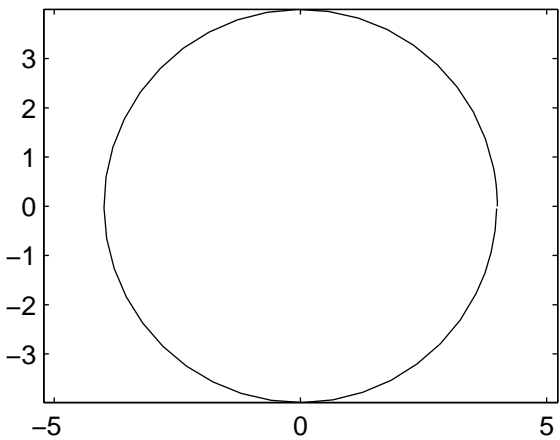
ode45: w(0)=.5
