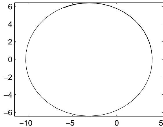
ode45: w(0)=.6
